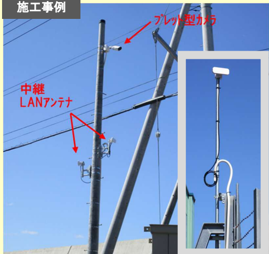
固定カメラと中継用無線アンテナ
