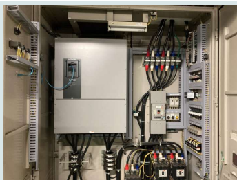
低圧汎用 インバータ盤 160KW
