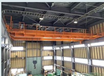
40 t ホイスト式天井クレーン
