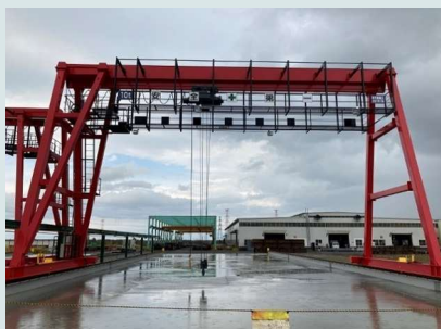
10 t 門型クレーン
